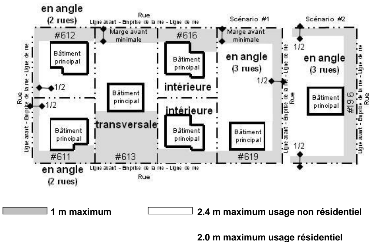
Figure 17.1 : Hauteur maximale des clôtures
